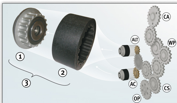
Рисунок 1: Шкив генератора с обгонной муфтой с гибкой соединительной муфтой и шестеренчатый привод.
