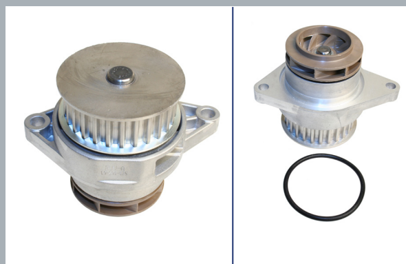
Рис. 1: Водяной насос 65468 старой конструкции
